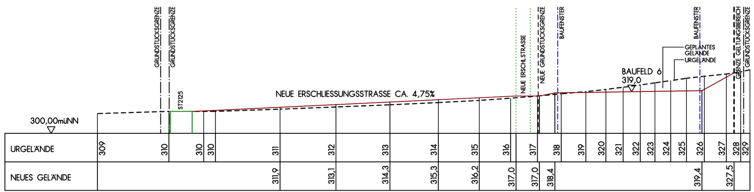
SCHNITT 3-3 M 1:1000/1000
