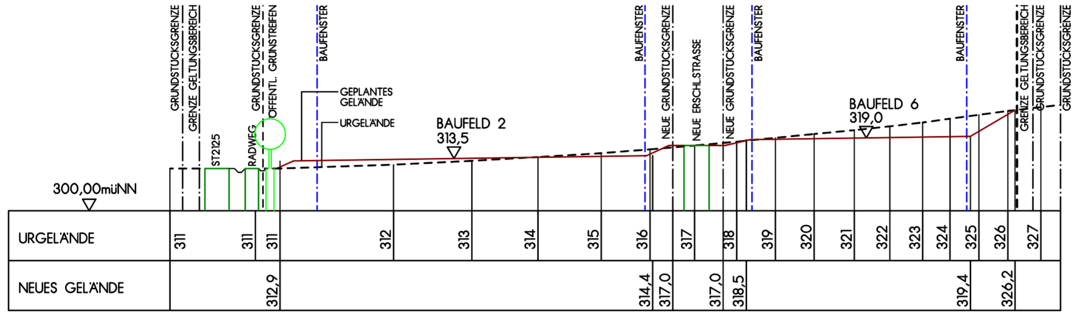
SCHNITT 2-2 M 1:1000/1000
