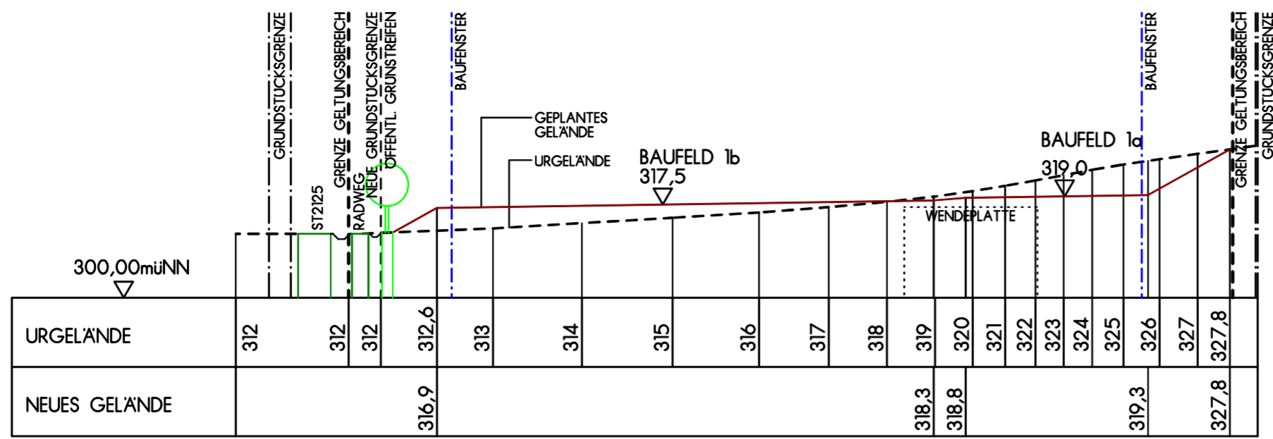
SCHNITT 1-1 M 1:1000/1000
