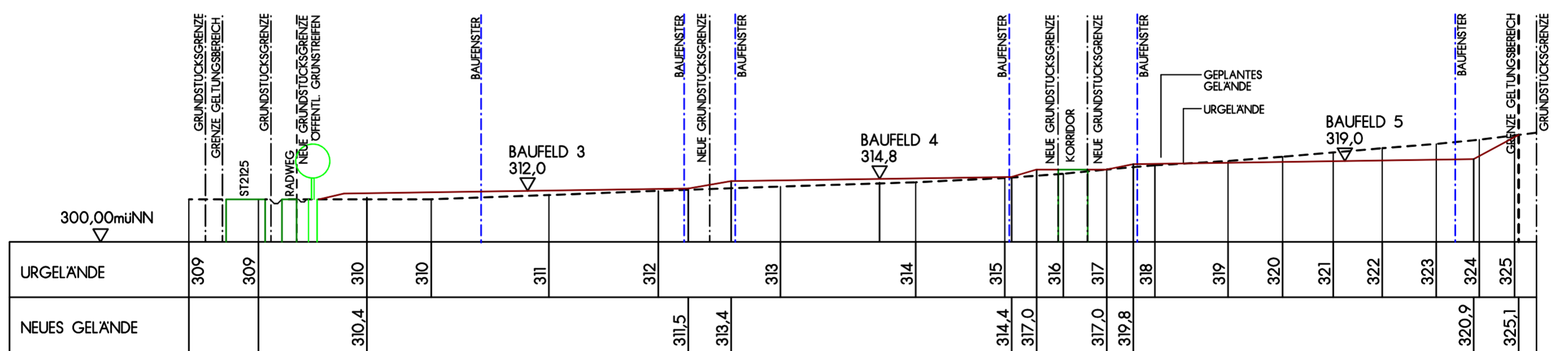
SCHNITT 4-4 M 1:1000/1000
